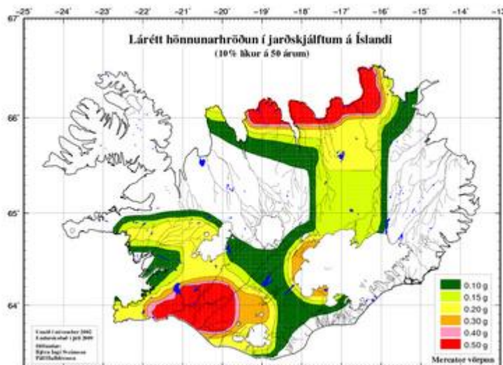
Mynd 43. Skipting Íslands í hönnunarhröðunarsvæði miðað við 500 ára meðalendurkomutíma. Heimild: Staðlaráð Íslands, Íslenskur staðall.
